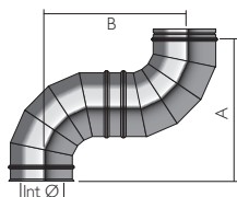
90° Offset
