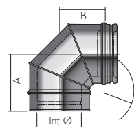
87° Bend
