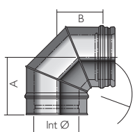
90° Bend
